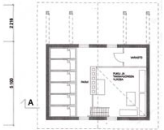
Ylävasen: Saunan alakerran pohjakartta Yläoikea: Saunan yläkerran pohjakartta Vasemmalla: Saunan läpileikkaus Huomatkaa etenkin lisätty terassi.
